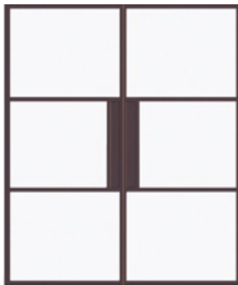
Rigel
